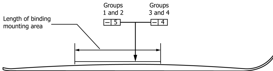
FIG. 1 Longitudinal Profile
