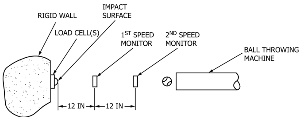
FIG. 1 Test Apparatus
