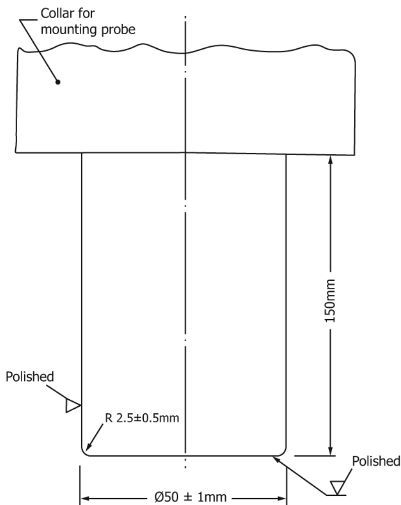
FIG. 1 Probe
