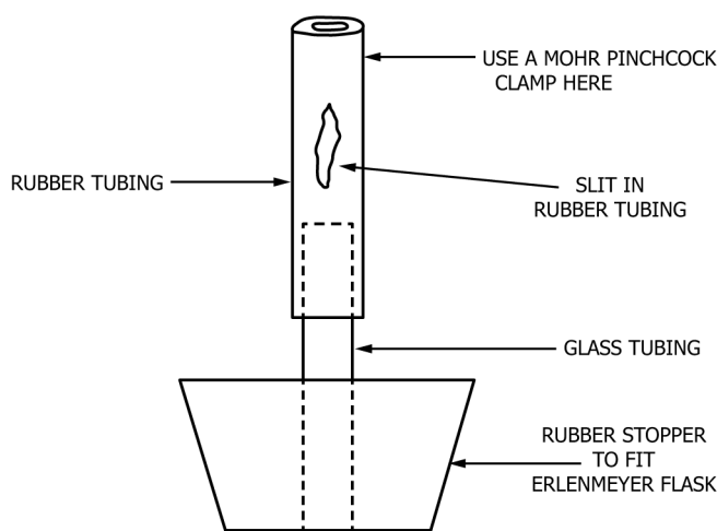
FIG. 1 Apparatus
