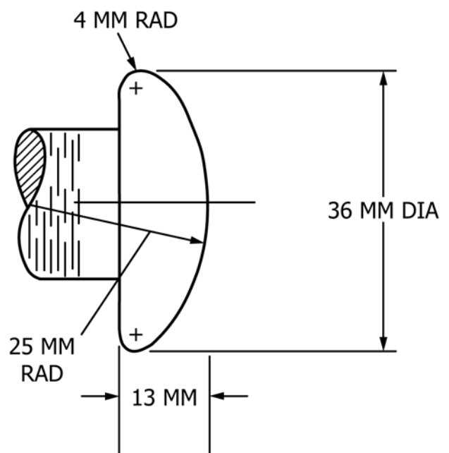
FIG. 1 VDE Electrode
