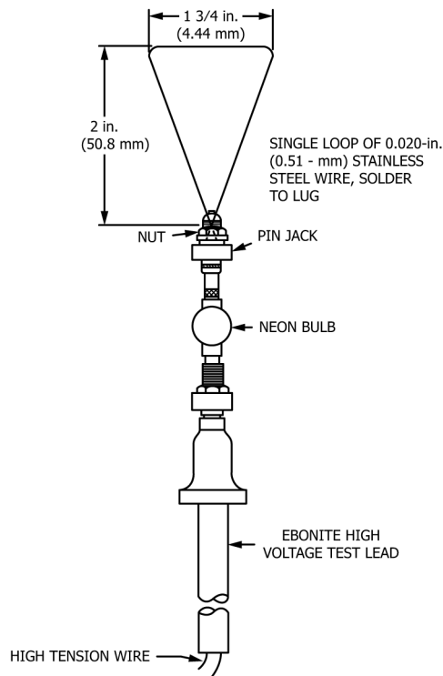
FIG. 1 Feeler
